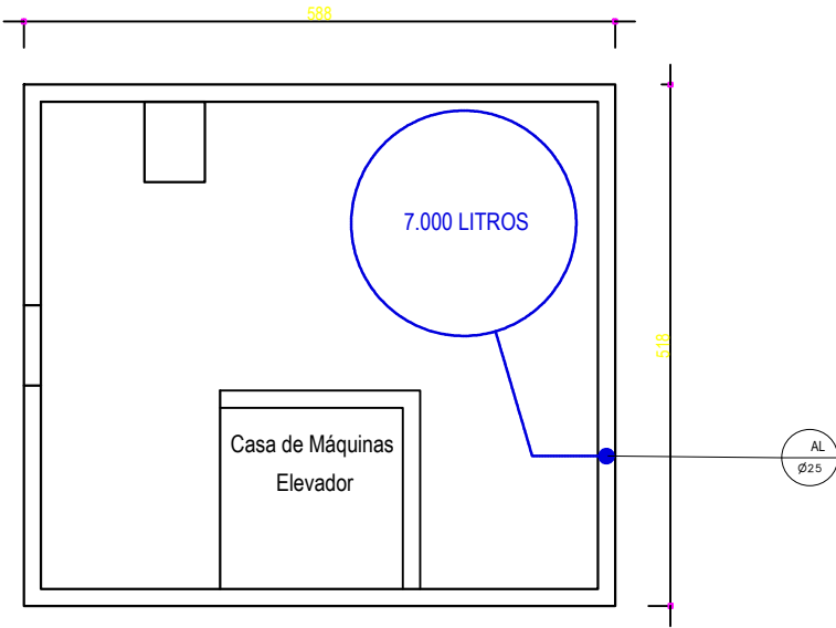
Casa de Máquinas Esc. 1/75
