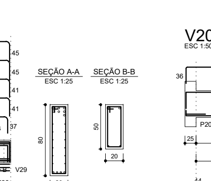
V20 ESC 1:50
