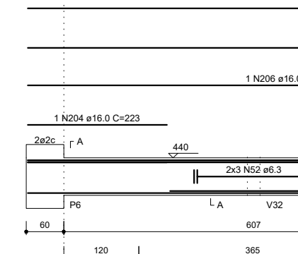
V3 ESC 1:50
