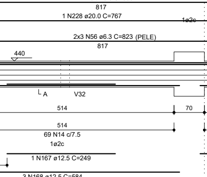
V7 ESC 1:50
