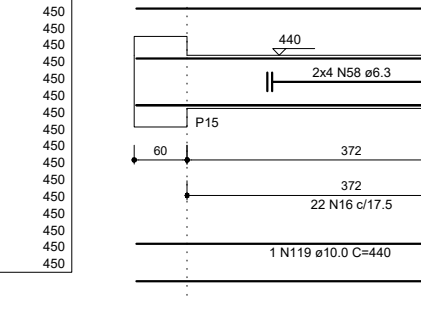
V11 ESC 1:50
