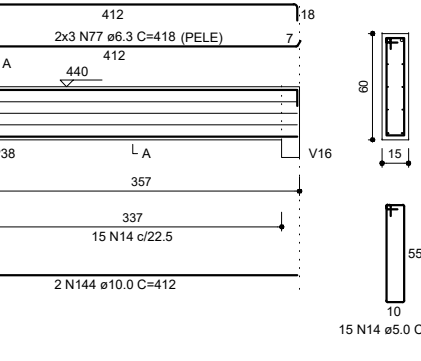
V23 ESC 1:50
