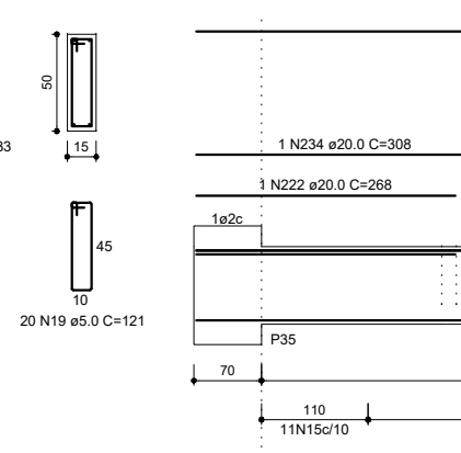
V15 ESC 1:50
