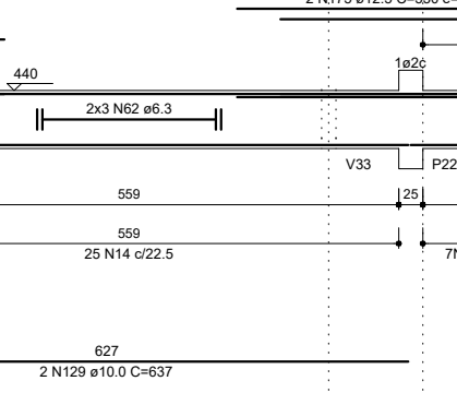
V13 ESC 1:50
