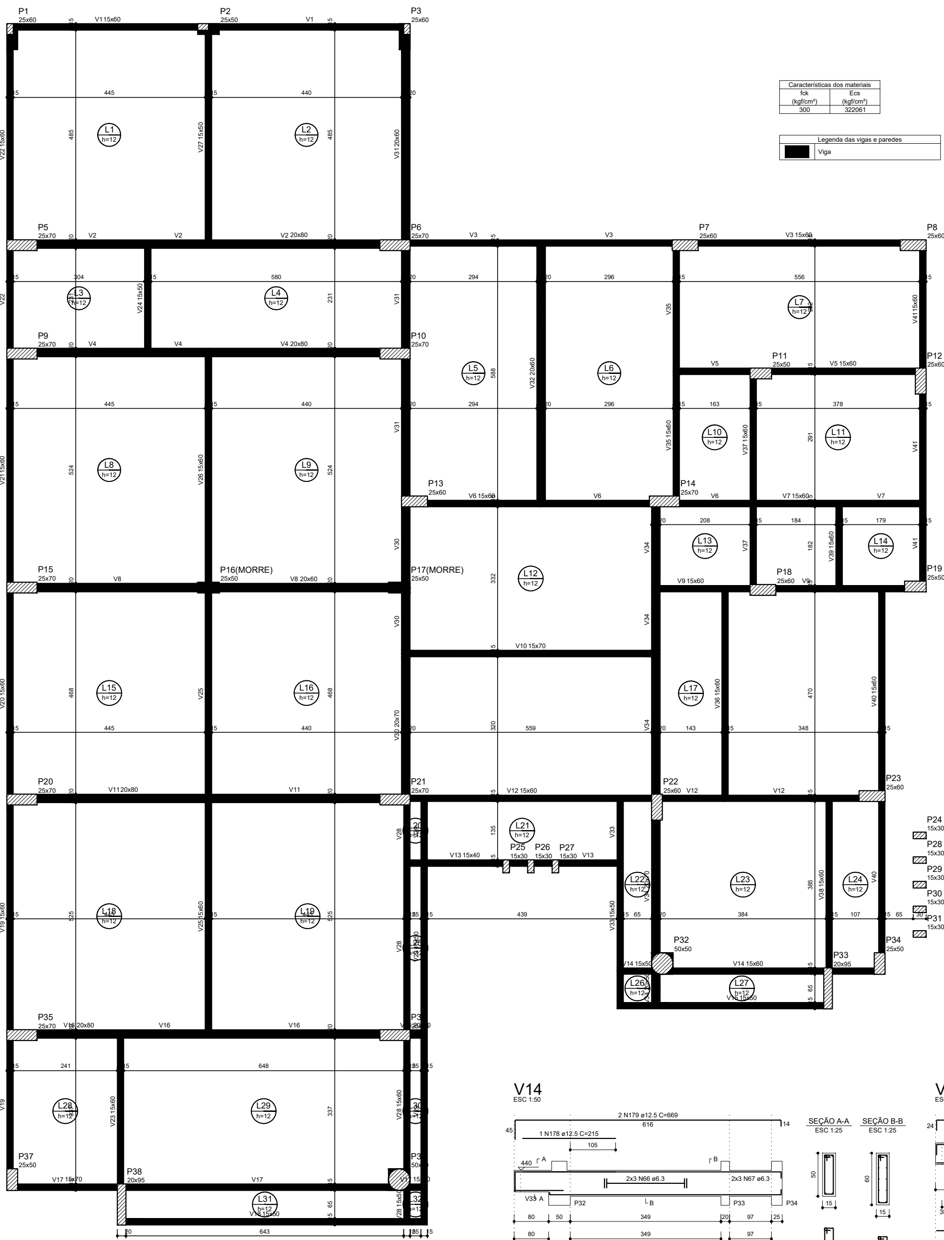
Forma do pavimento Entre Pisos (Nível 440) escala 1:50
