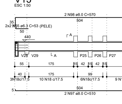
V10 ESC 1:50
