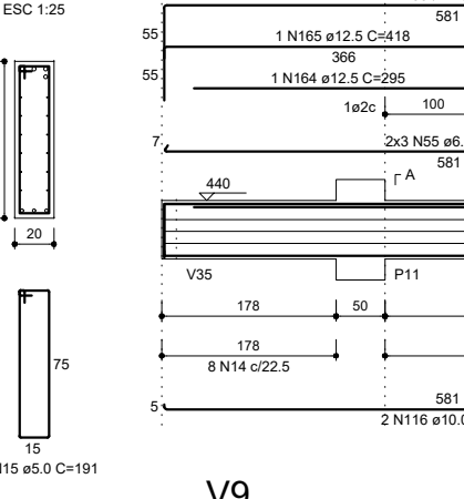
V9 ESC 1:50
