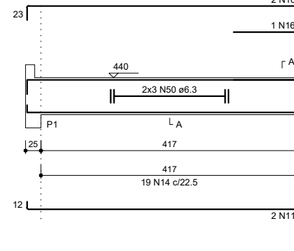
V1 ESC 1:50
